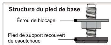
1. Lors de la palpation de la machine, vérifiez si le pied inférieur est à l'état d'usine. Sinon, veuillez remettre le pied inférieur à l'état d'usine : l'écrou de blocage est fermement verrouillé sur le fond de la boîte, et le pied de support est fermement verrouillé sur l'écrou de blocage.
